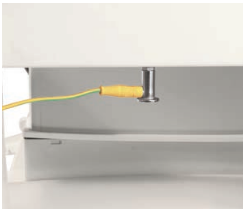
Equipotential Cable Link AC968A
